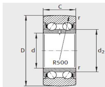
LR52...-2Z、 LR53...-2Z、 LR52...-X-2Z 1)
