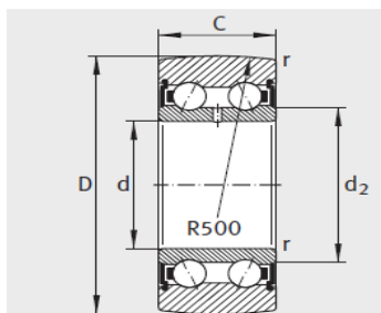
LR50...-2RS、 LR52...-2RS、 LR53...-2RS
